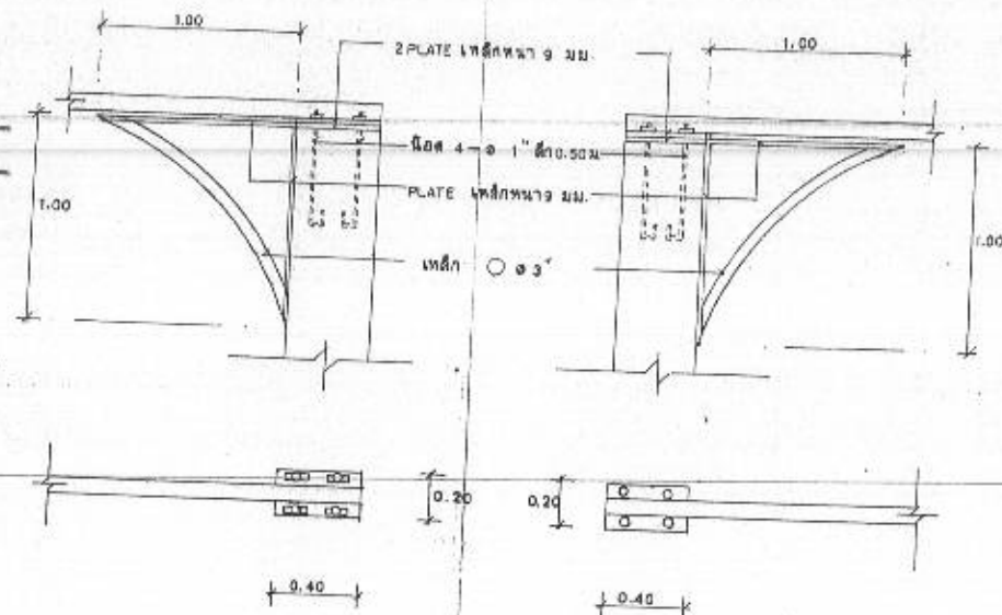
ขนาดหน้าแปลน 1:20 ขนาดหน้าแปลน 1:20
