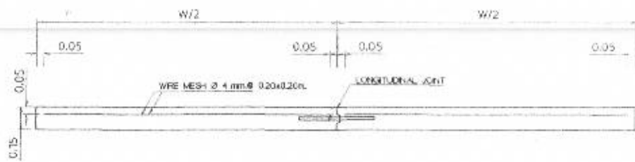
รูปตัดตามขวางตัวจราจร ค.ส.ฉ. Scale 1:25
